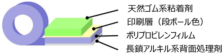
図. No.3523 テープ構成
